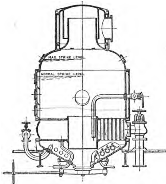
FIG. 28.—CALANDRIA-PAN 1
